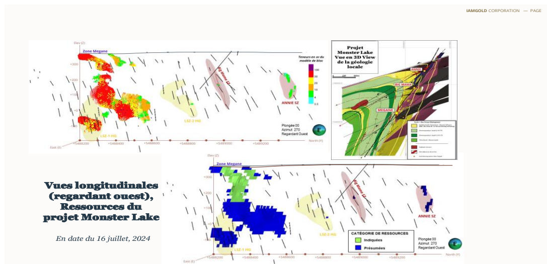
Figure 4 : Sections longitudinales de Monster Lake – Modèles de blocs des ressources de la zone Mégane comportant une distribution des teneurs en or et des volumes de contraintes sous terre (DSO).
