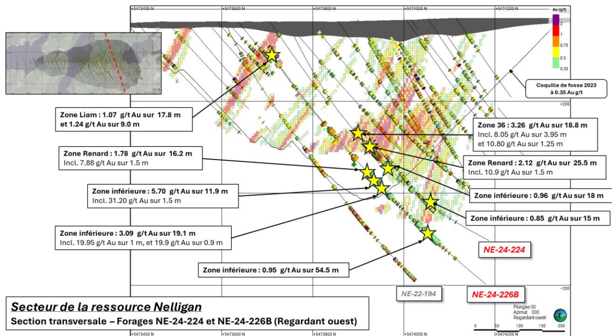
Figure 3 – Section transversale – Forages NE-24-224 et NE-24-226B (Regardant ouest)
