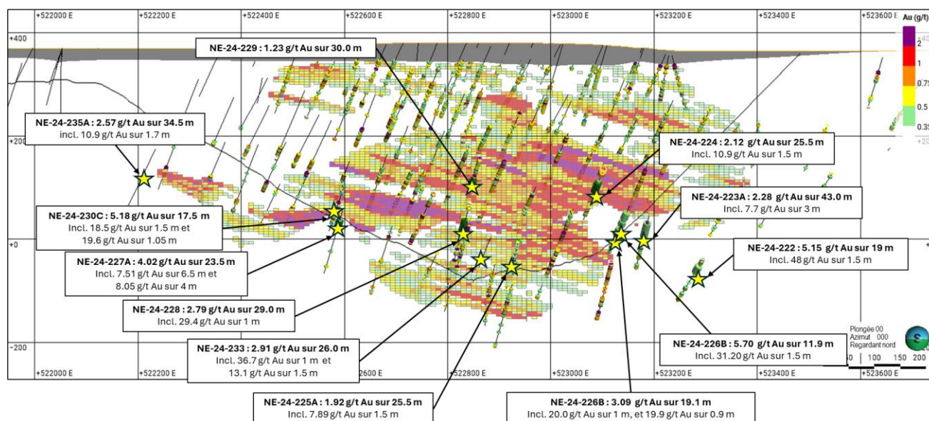
Figure 2 – Section verticale longitudinale de la zone Renard et de la zone inférieure
