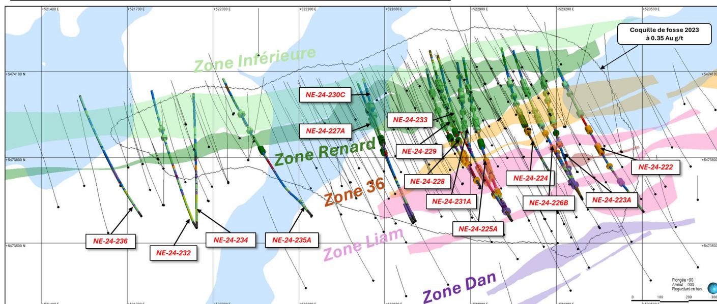
Figure 1 – Plan de surface des trous de forage
